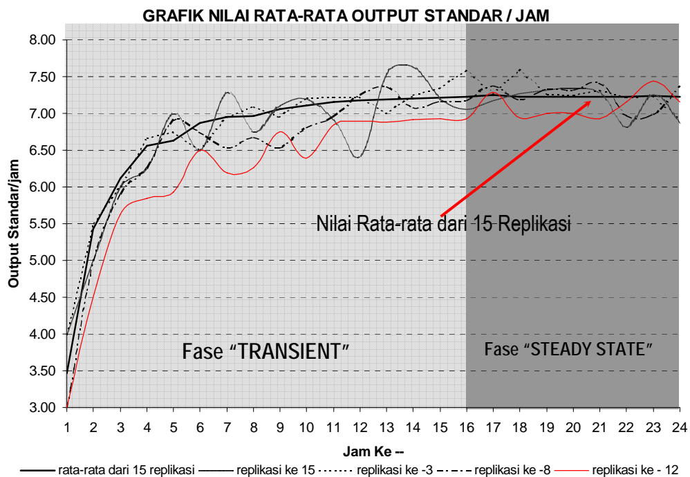
Gambar 5. Estimasi Fase “STEADY STATE” Pada model Simulasi
