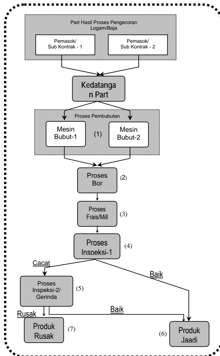
Gambar 1. Aliran Proses Sistem Produksi yang diamati
